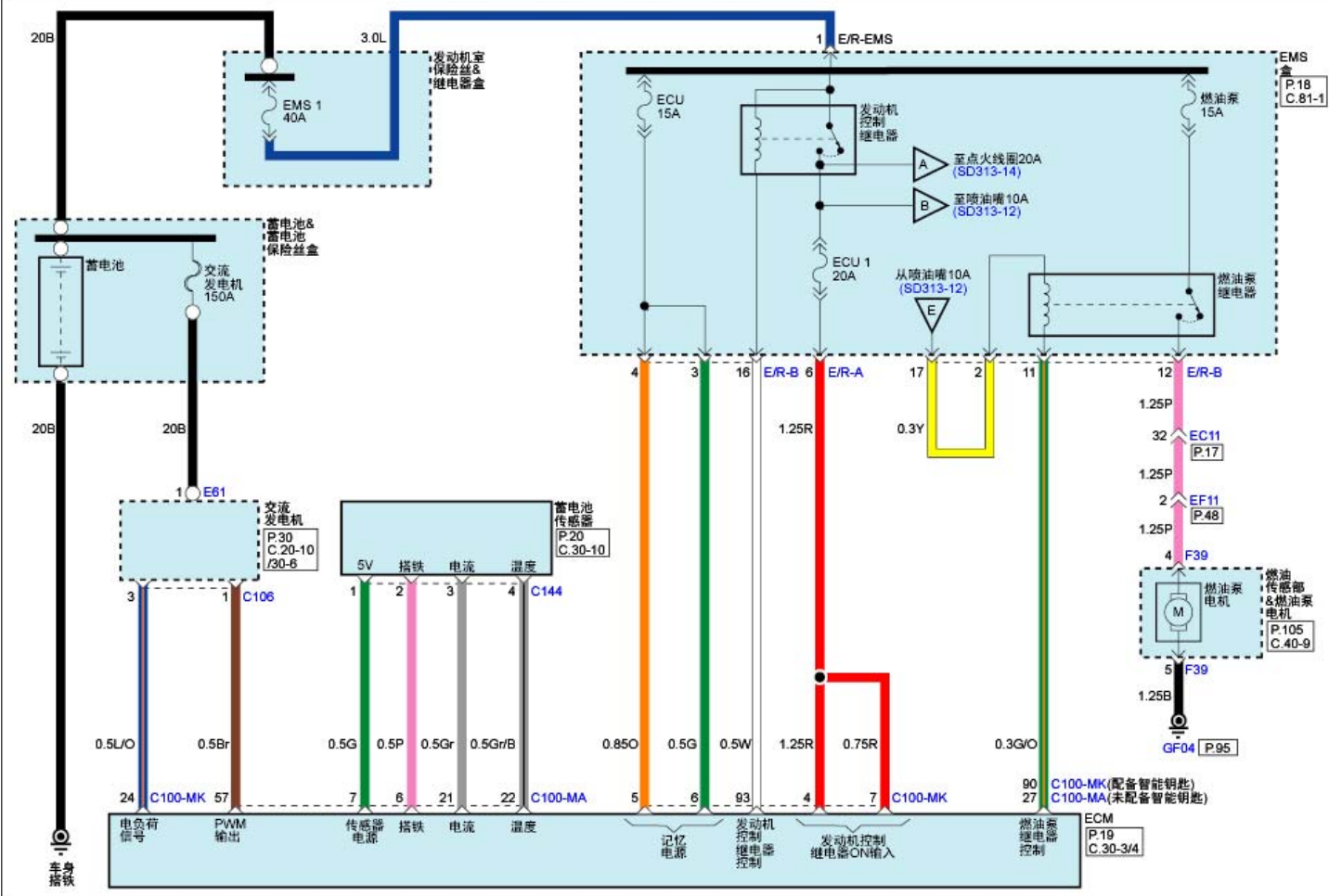
发动机控制系统(G4NB/G4NA : NU 1.8L/2.0L MPI M/T)(3)
